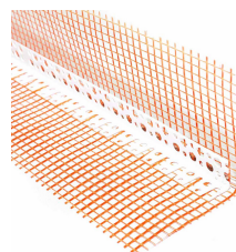
PROFIL COLT CU PLASA, PVC, 200 X 200 X 3000 MM
