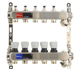
KIT DISTRIBUITOR CALORIFERE, 1"-3/4, 5 CAI, CU ROBINET
